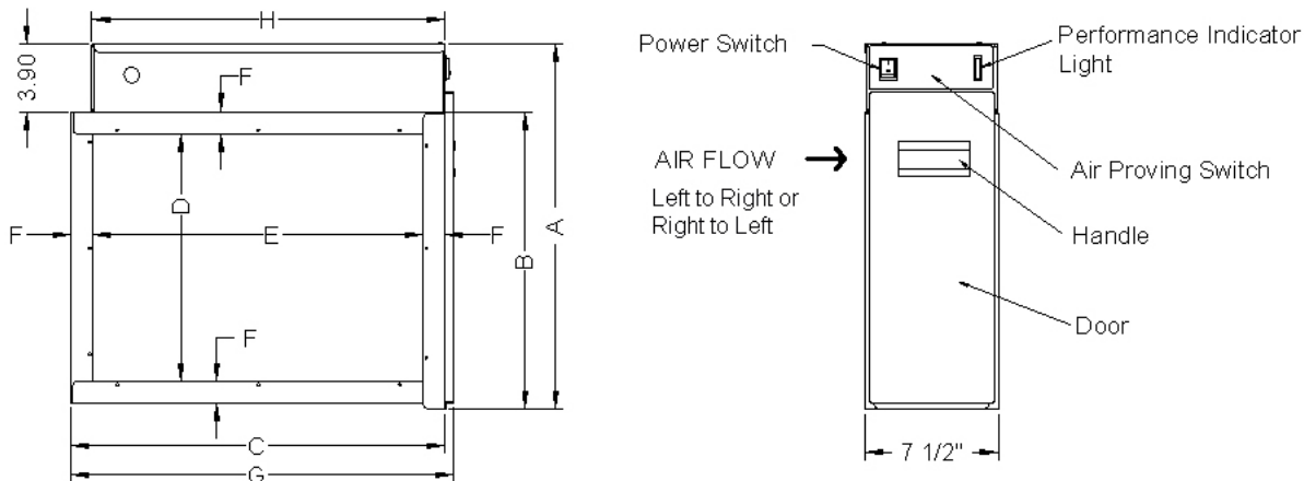
Fig. 3 — DIMENSIONS
